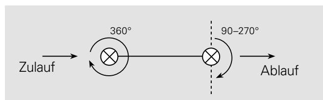
Draufsicht: Zulässiger Winkel des Zu- und Ablaufes
