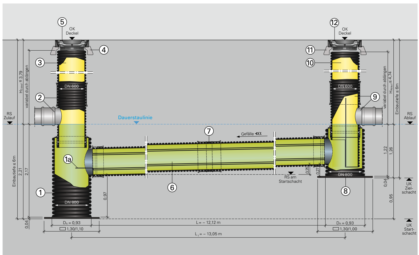
Längsschnitt SediPipe L plus 600/12
