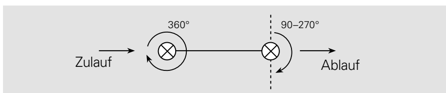
Draufsicht: Zulässiger Winkel des Zu- und Ablaufes
